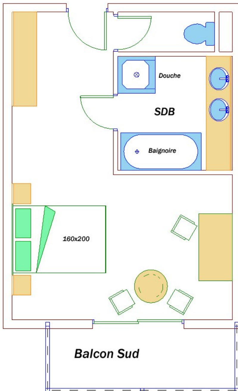
«Savoyard» (35m 2 )
